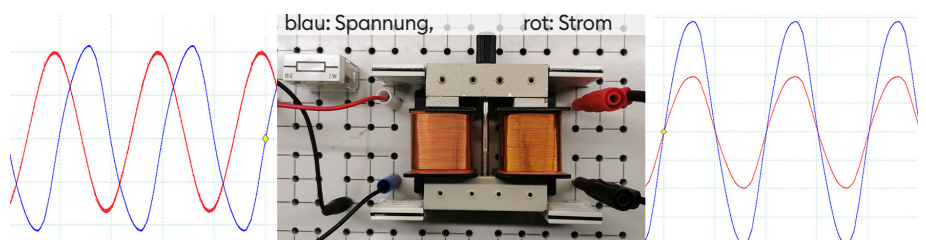
Bild 3: Der Versuchsaufbau und die Bilder des Oszilloskops zeigen die grundsätzliche Transformatorschaltung mit dem primär- und sekundärseitigen Spannungs- und Stromverlauf bei Sinusbetrieb.
