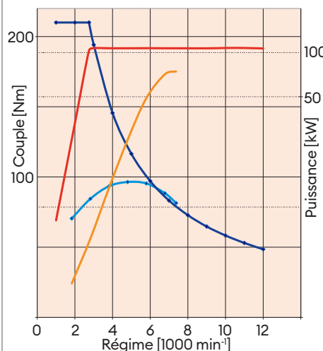
Diagramme puissance-couple.
