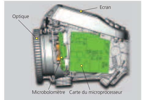
Fig. 5. Structure d'une caméra FLIR.
