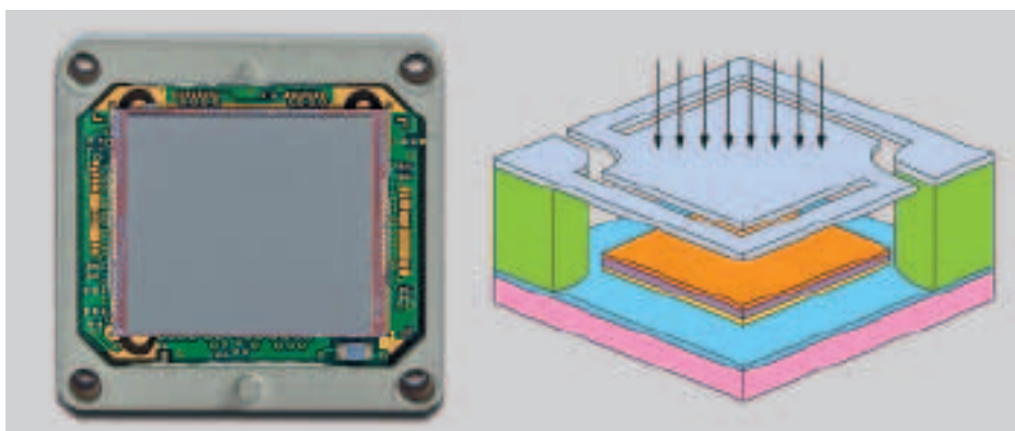
Fig. 4. A gauche, le tout nouveau microbolomètre «Muon» de FLIR. A droite, un élément résistif individuel responsable d'un point d'image.
