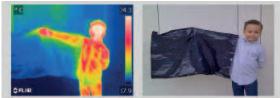
Fig. 3. Le rayonnement thermique est visible avec la caméra infrarouge, également au travers d'un sac en plastique noir.
