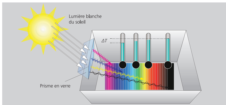
Fig. 1. L'expérience réalisée par Herschel démontre que la température augmente dans la plage des rayons infrarouges.
