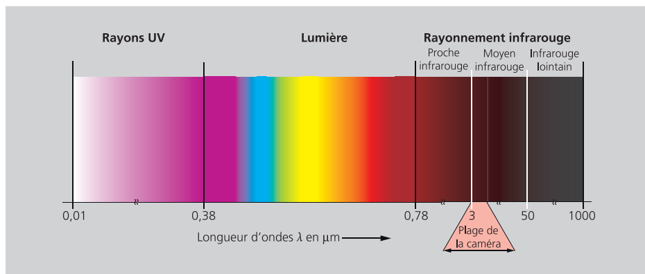
Fig. 2. Le rayonnement infrarouge utilise une partie du spectre électromagnétique.
